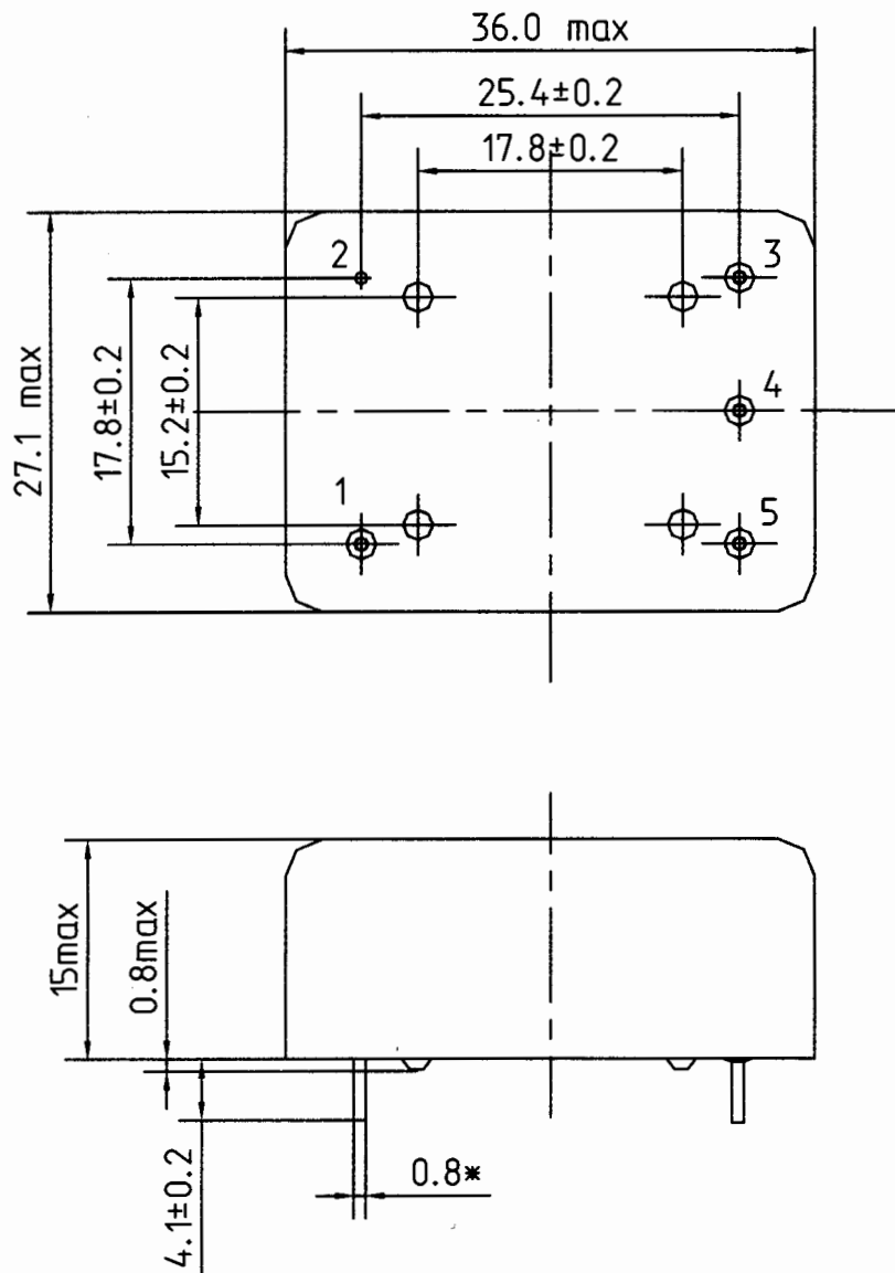
маркировка выводов может отсутствовать Рисунок 1
